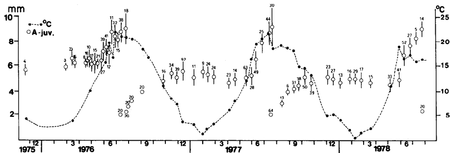
Abb. 5: Wassertemperatur im Flemhuder See und durchschnittliche Größe der jeweils jüngsten Generation von Cyathura carinata (senkrechte Linien = Standardabweichung, darüber oder darunter Individuenzahl)
