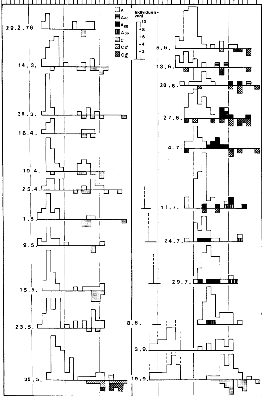
Abb. 4: Absolute Zahl und Länge der Stadien von Cyathura carinata in den Proben aus dem Flehmüder See. A: Jungtiere und unreife ♀, A oo : ♀ nach der Parturialhäutung, A oo- : bruttragende ♀, A oo- : ♀ mit entleertem Marsupium, C: Vormännchen, C♂: Vormännchen mit appendix masculina und ohne Aesthetaskenbüschel an der 1. Antenne, C♂: geschlechtsreife ♂ mit Aesthetaskenbüschel
