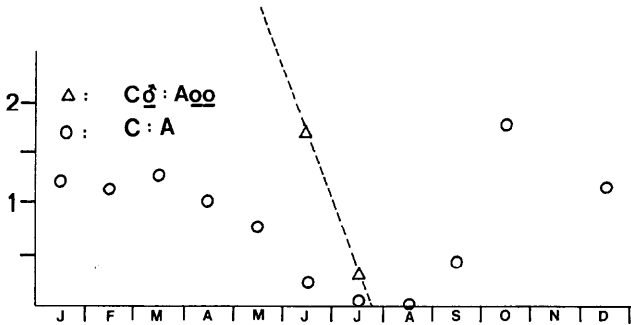
Abb. 9: Verlauf des C_3\delta : A_{00} - (geschlechtsreife Tiere) und des C:A - Quotienten (unreife Tiere), Summe aus 3 Brutperioden
